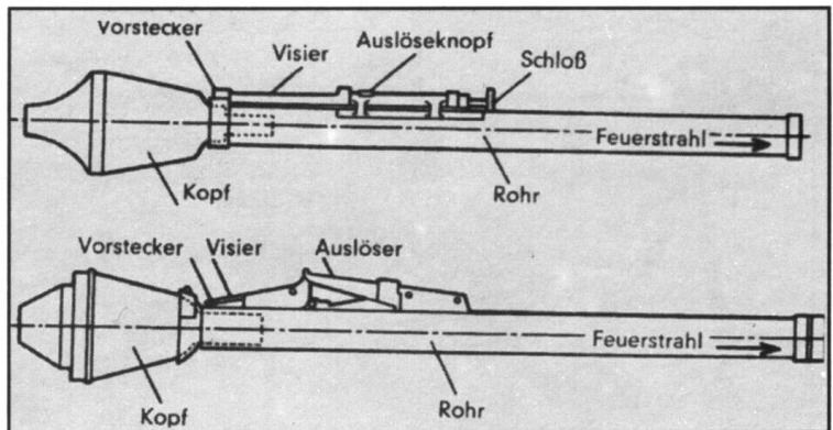
Панцерфауст 30 (вверху), панцерфауст 100 (внизу), слева - гранатер, вооруженный панцерфаустом 100
